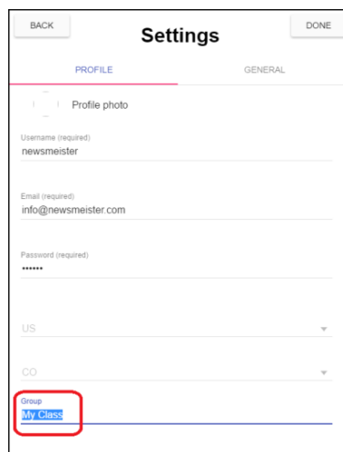
Web Version
